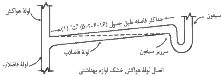
شکل شماره (۱۶-۶-۲-۵) "ت": اتصال لوله هواکش خشک لوازم بهداشتی
