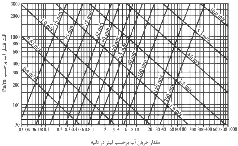
شکل پ ۵-۱-۸ (SI) منحنی اندازه گذاری لوله‌های پلاستیکی
