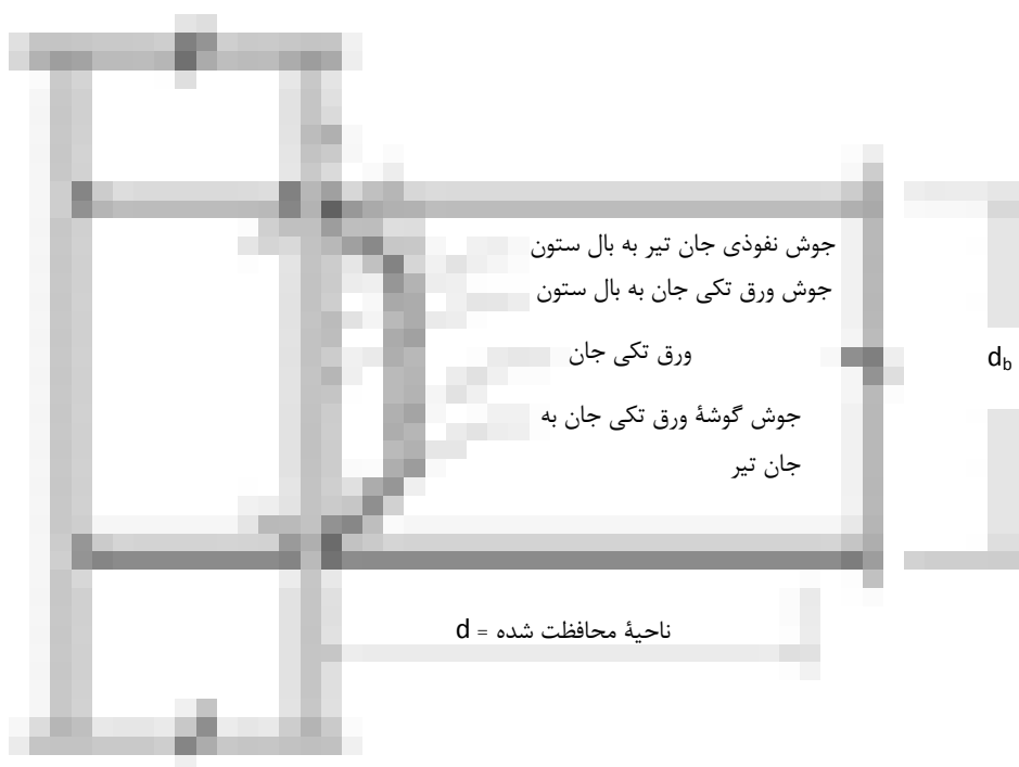
شکل ۱۰-۳-۱۳-۵ اتصال گیردار تقویت نشده جوشی (WUF-W)
