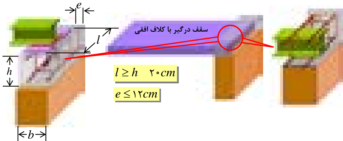
شکل پ-۲-۹- جزئیات اتصال سقف طاق ضربی با کلاف افقی و دیوار بار بر
