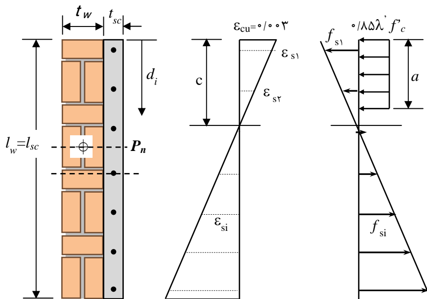
شکل ۶-۱- مقطع دیوار یکطرفه تقویت شده با پوشش بتن مسلح
