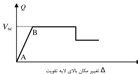
شکل ۶-۴- منحنی عمومی رفتار غیرخطی لایه تقویت
