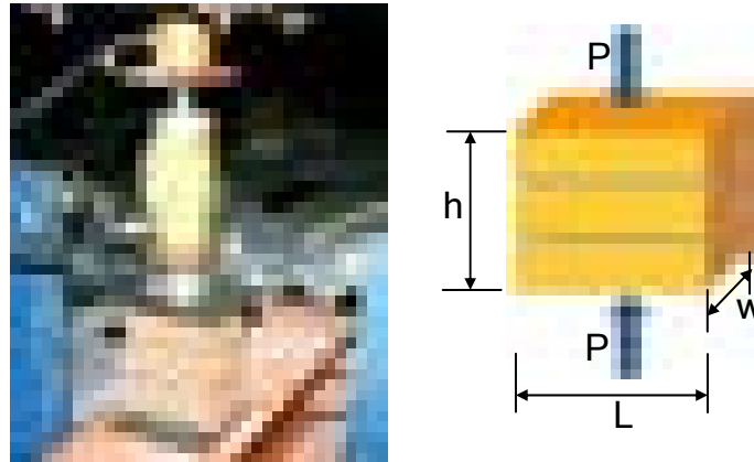
شکل ۲-۲- نحوه انجام آزمایش منشور آجری در آزمایشگاه
