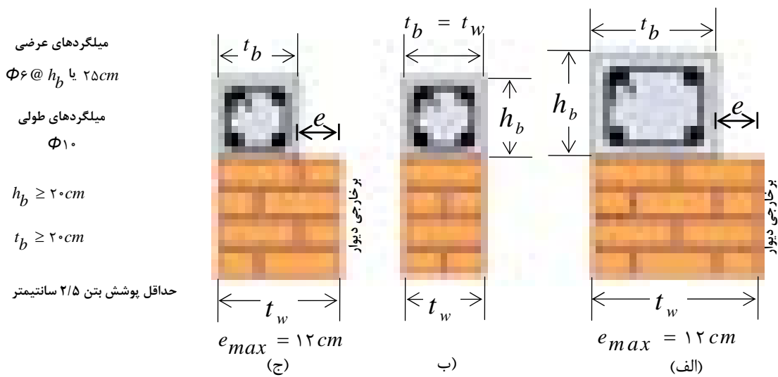
شکل پ-۲-۲۲- نحوه اجرای صحیح کلاف افقی روی دیوارهای بار بر
