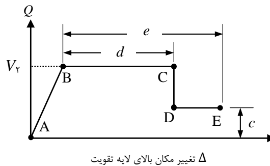
شکل ۶-۳- منحنی رفتار غیرخطی لایه تقویت براساس تغییرمکان نسبی
