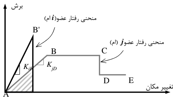
شکل ۴-۵- منحنی رفتاری عضو تغییرشکل-کنترل و نیرو-کنترل
