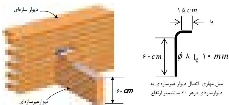
شکل پ-۲-۴- نحوه درگیر کردن دیوار غیر سازه‌ای به دیوار سازه‌ای
