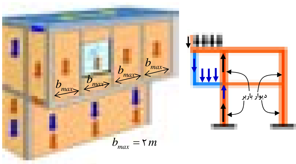
شکل پ-۲-۱۷- نحوه انتقال بار پیش آمدگی، بار سقف به دیوار زیرین
