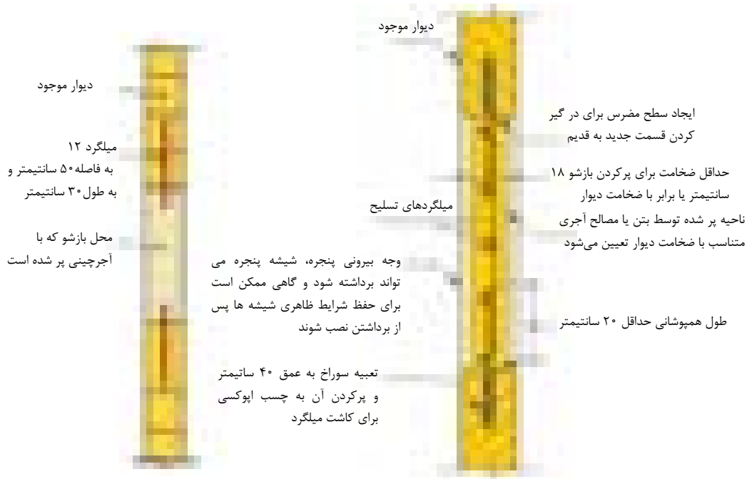
شکل ۵-۱۱- یکی از راه‌های کاهش ابعاد بازشوها
